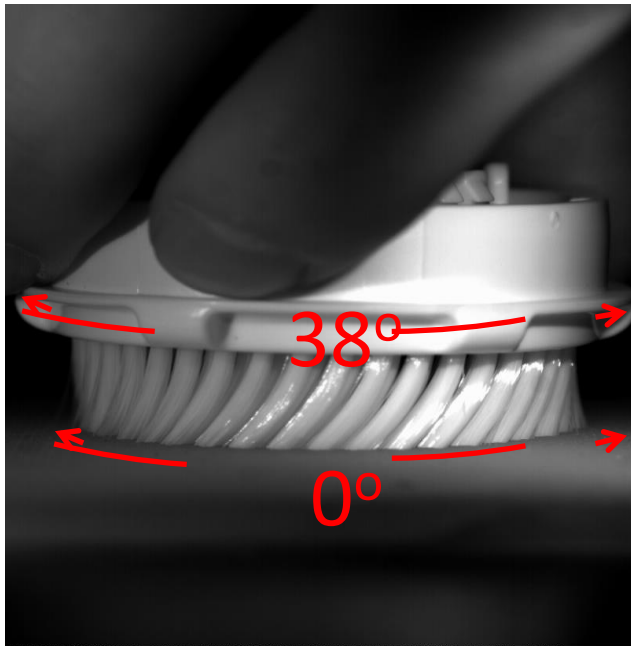
毛刷小角度轉動時 僅刷毛在彎曲
